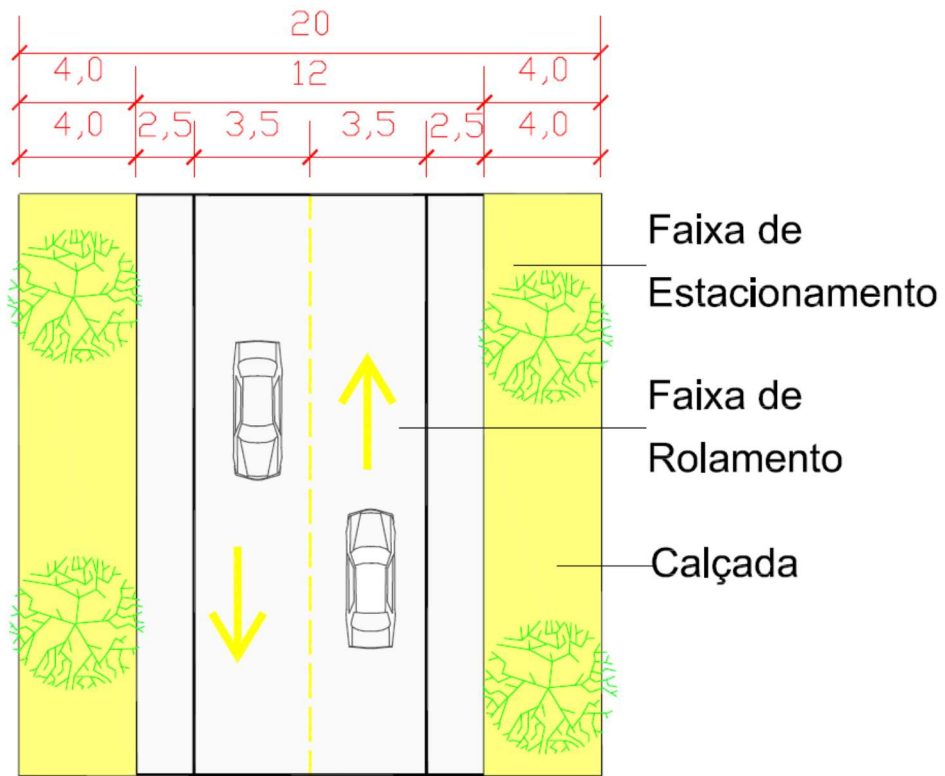
Planta Esquemática
