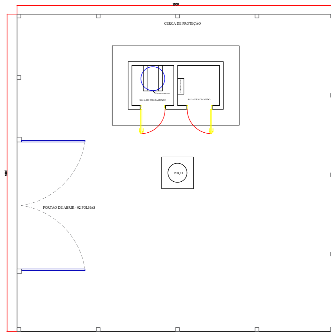
PLANTA DE SITUAÇÃO - CERCA DE PROTEÇÃO DA CASA E Escala 1/25
