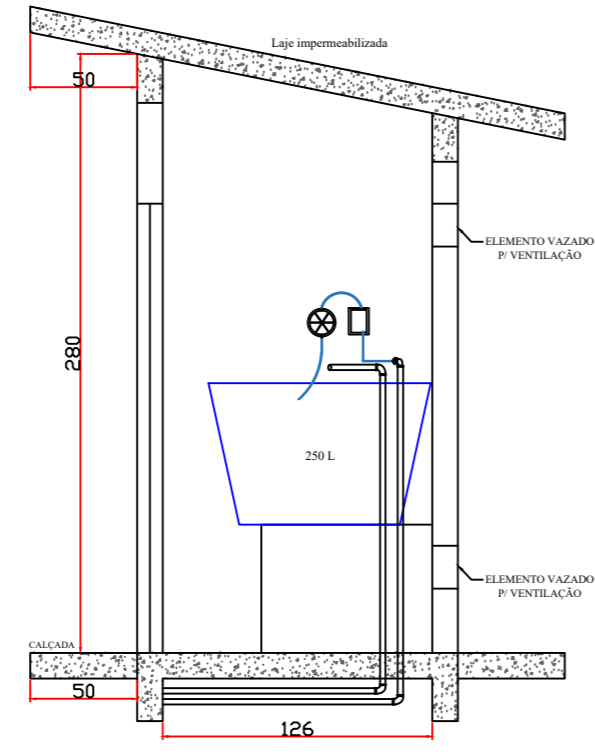
CORTE AA Escala 1/25
