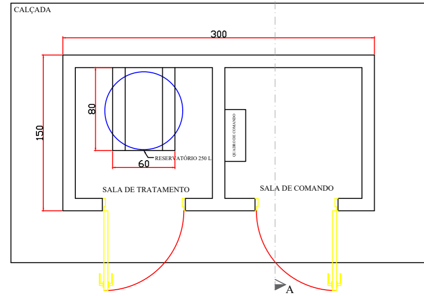
PLANTA BAIXA - Área= 4,50m 2 Escala 1/25
