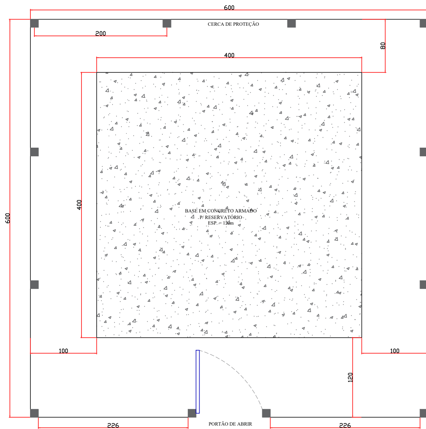
PLANTA BAIXA - RESERVATÓRIO Escala 1/25
