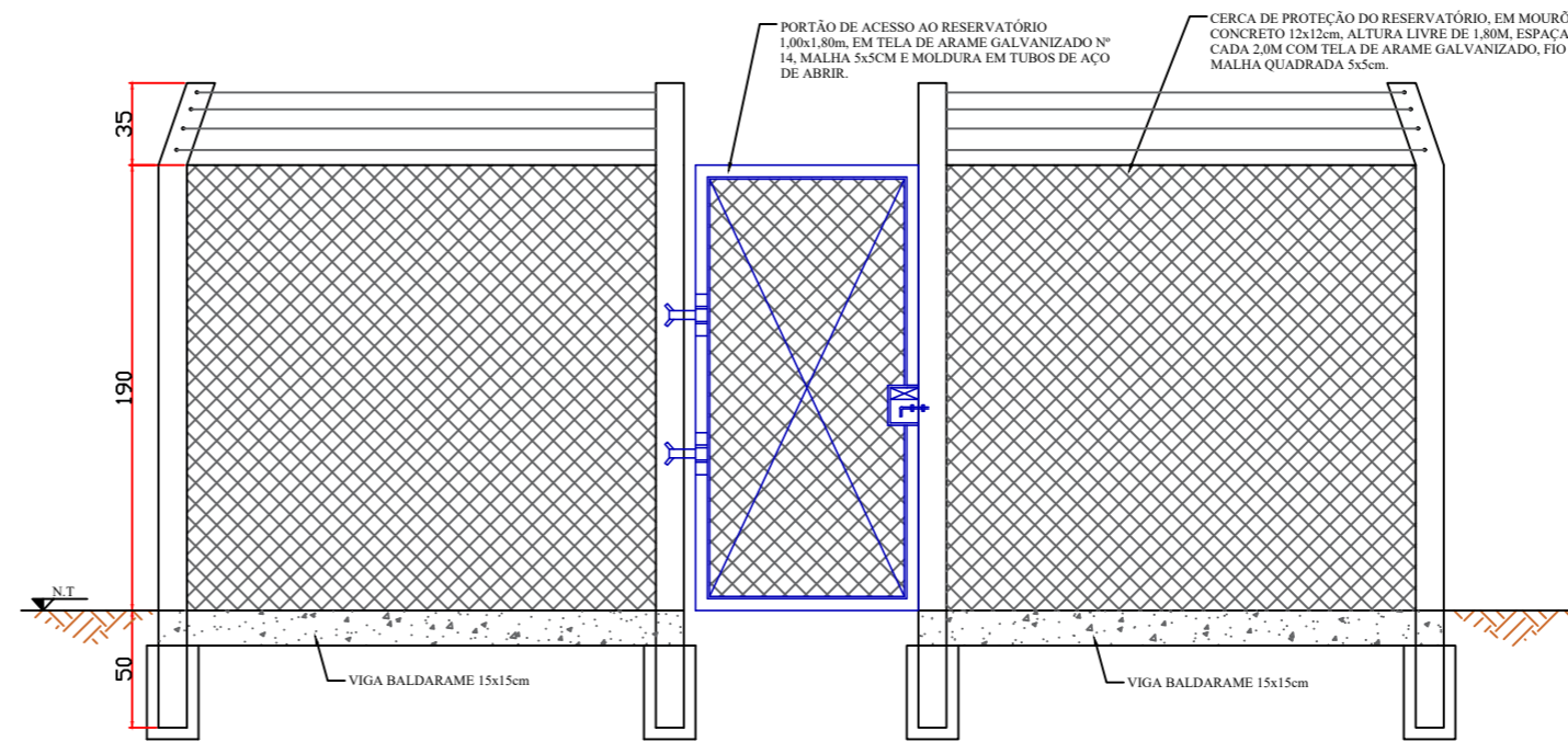
ELEVÇÃO FRONTAL - CERCA DE PROTEÇÃO PORTÃO RESERVATÓRIO Escala 1/25
